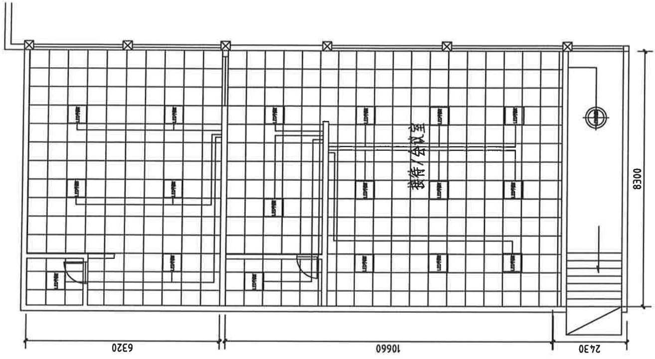
办公区天花、照明施工图
