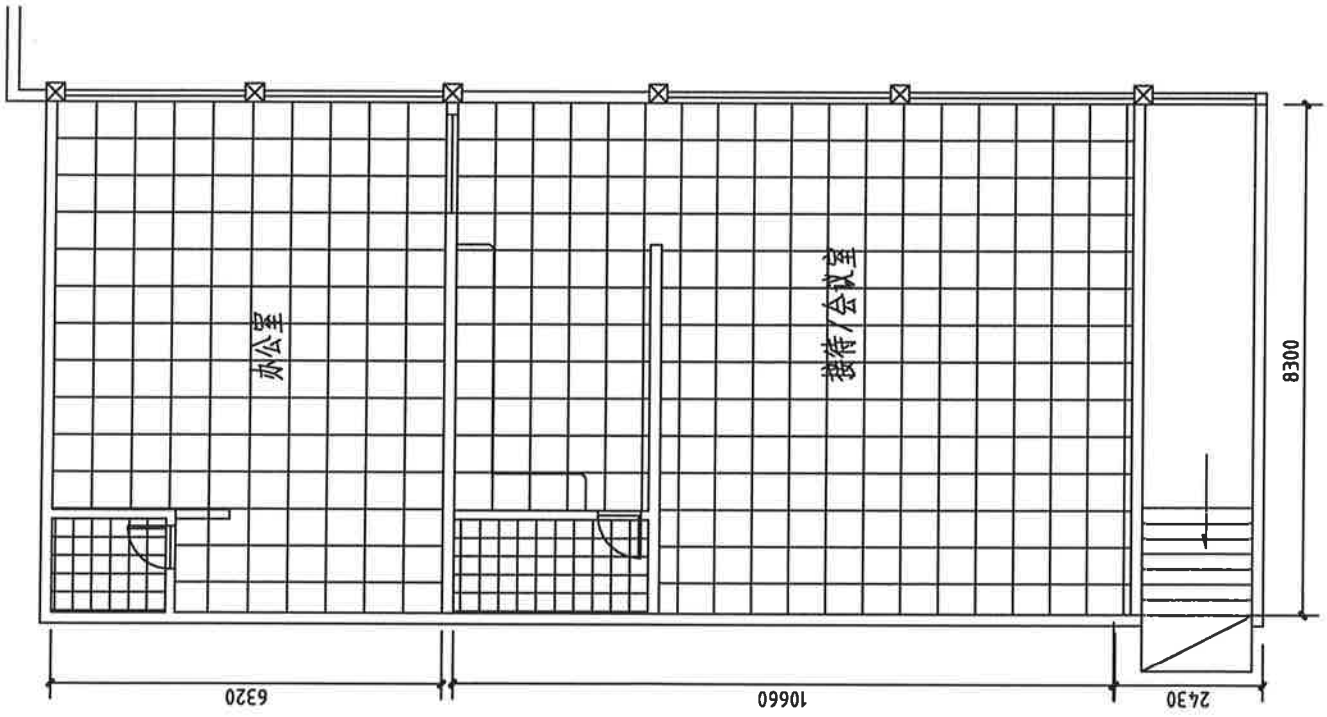
办公区地面施工图
